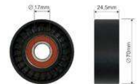
FT44556 STEUERUNGSSPANNER ROLLE
